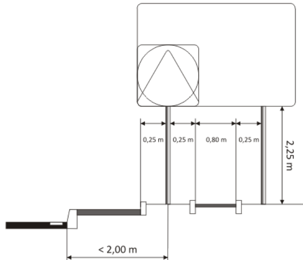
Slika 2: Postavitev znaka v naselju ob pločniku
