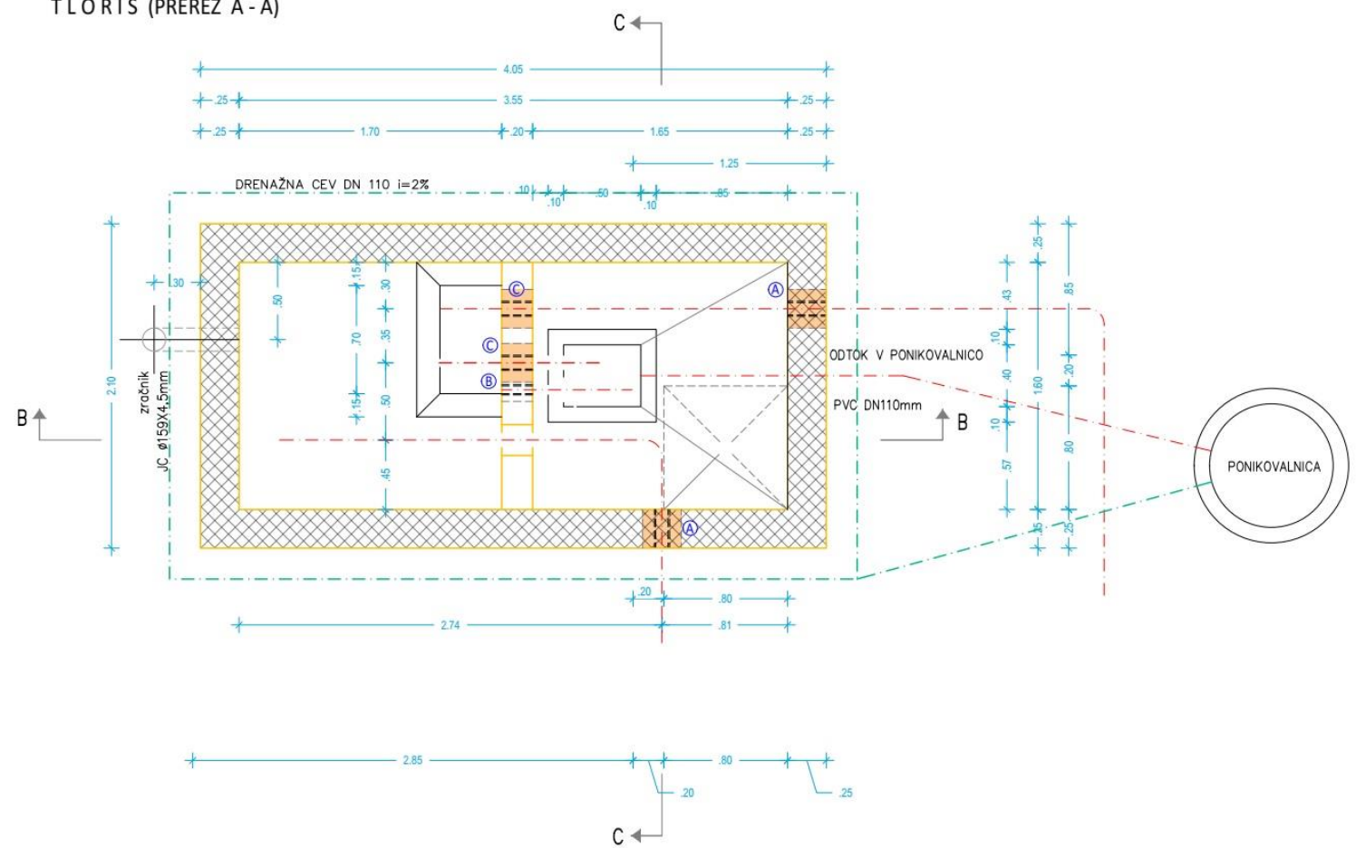
TLORIS (PREREZ A - A)
