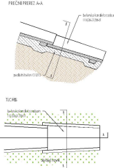
DETAL VGRAJEVANJA BETONSKE KANALETE IN MILDASTEGA POLJA M1:25
