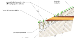
DETAL ITOČNE GLAVE M1:25
