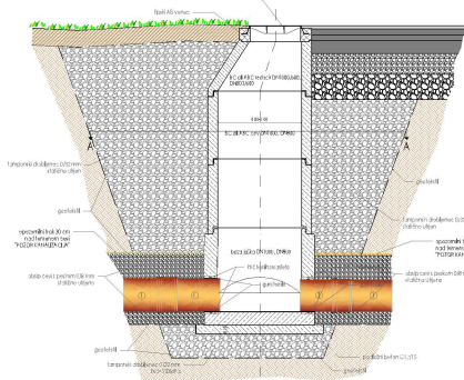
DETAL REVULSKEGA JAŠKA DN1000, DN800- TRAVNATE/ASFALNE POVRŠINE (FEK, MET) M1:25
