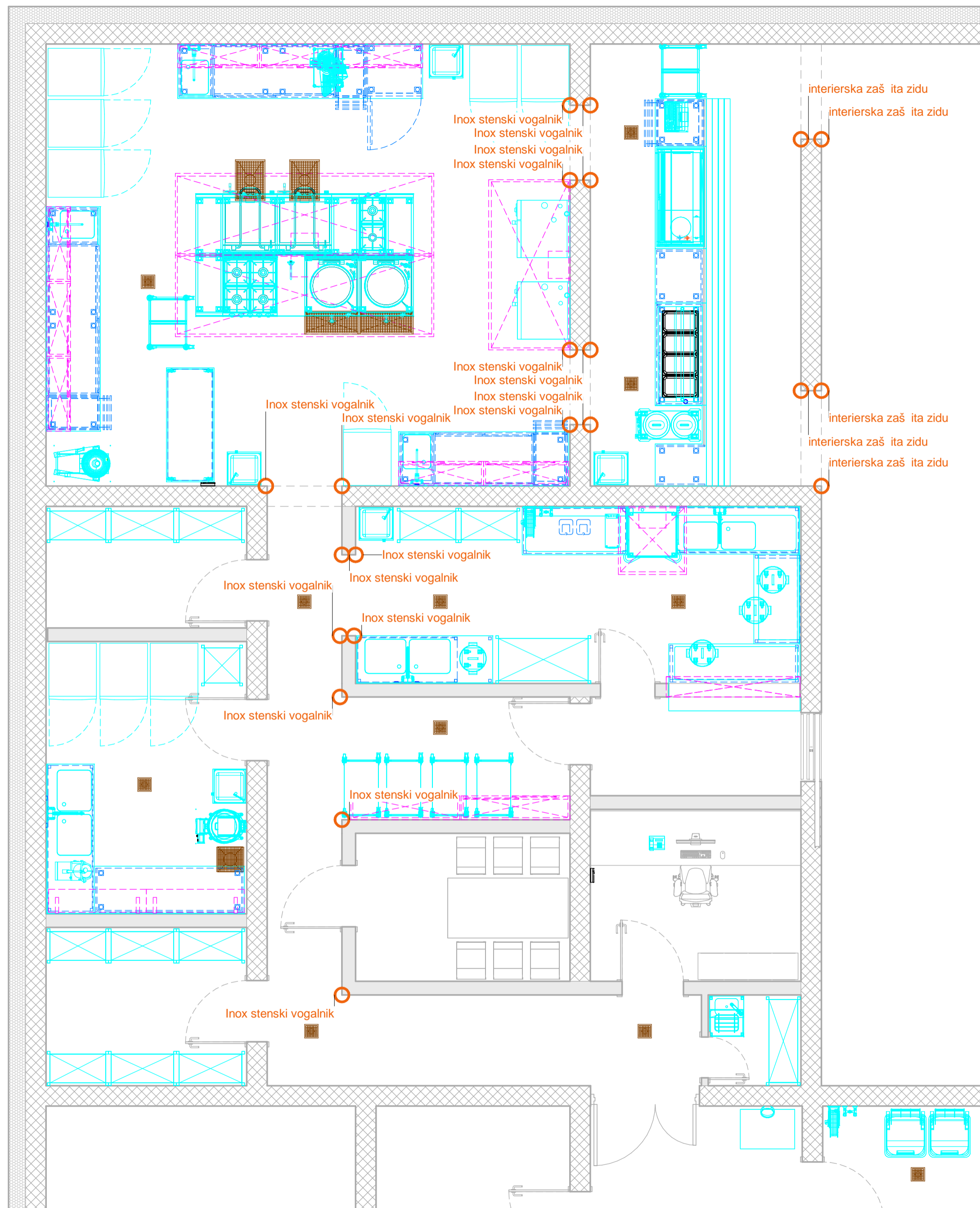
Risba pozicij stenskih vogalnikov M 1 : 50
