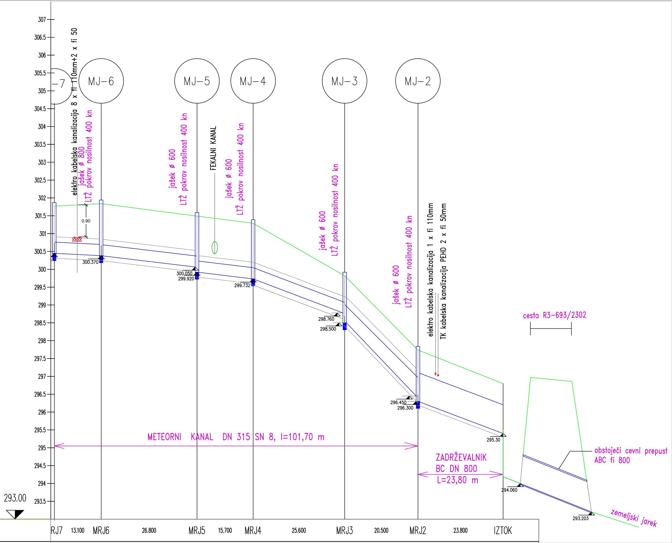
PROFIL-2: OS_METEORNI MEROLO 1:500/50
