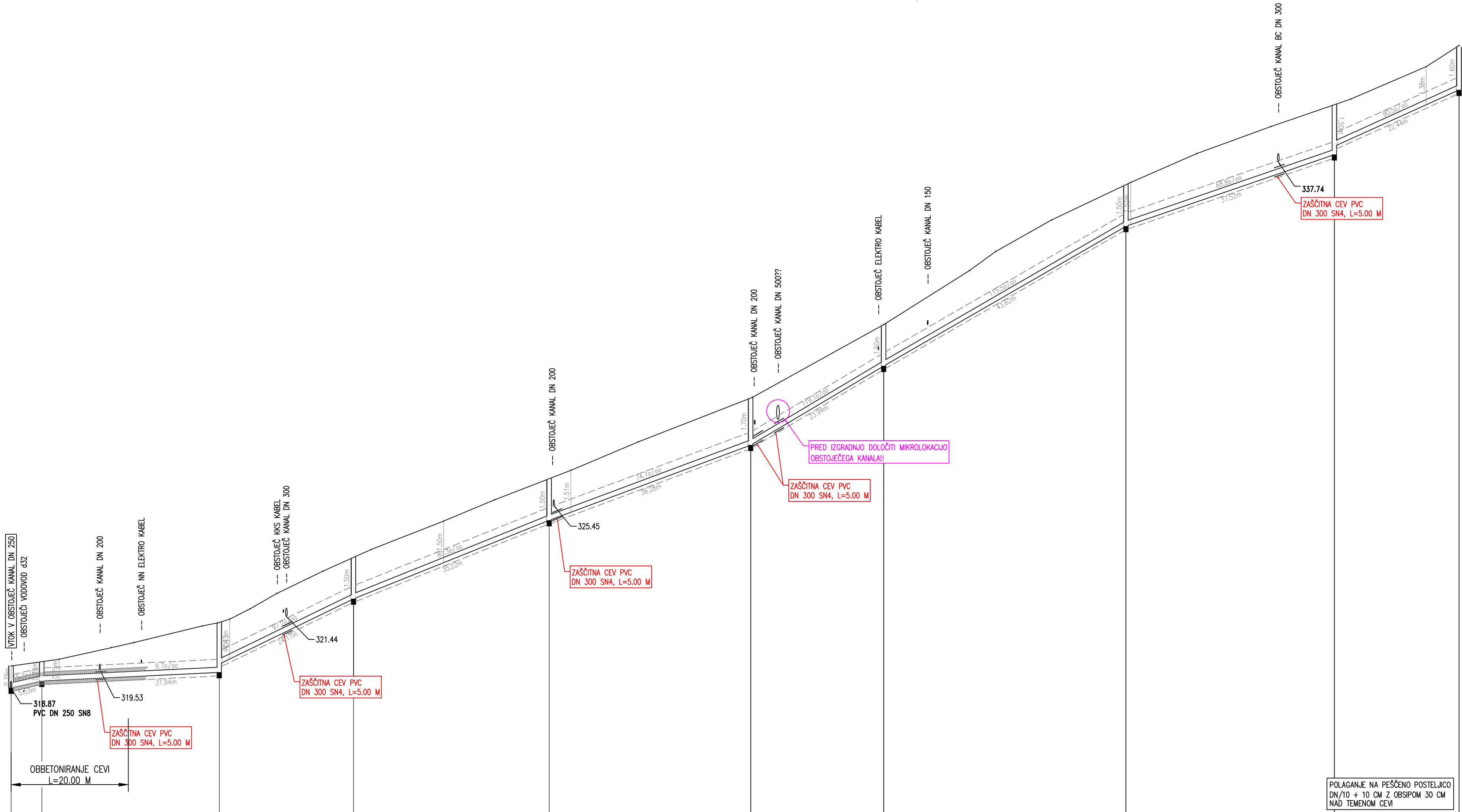
PODOLŽNI PROFIL FEKALNEGA KANALA 1.8 M 1:500/100
