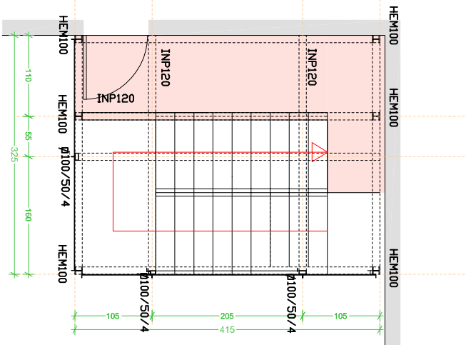
tloriš: POŽARNO STOPNIŠČE - mansarda
