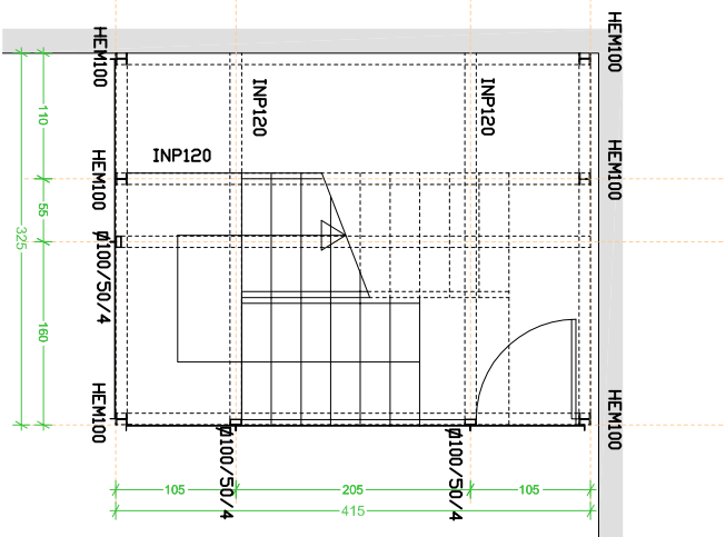
tloriš: POŽARNO STOPNIŠČE - v prilježju
