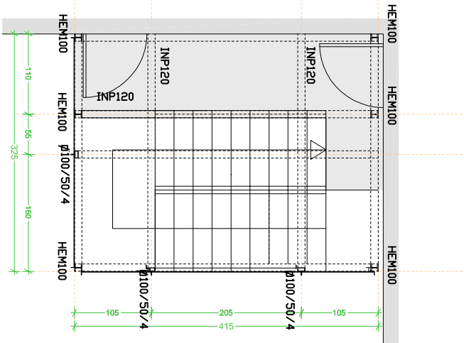
tloriš: POŽARNO STOPNIŠČE - etaža pod mansardo
