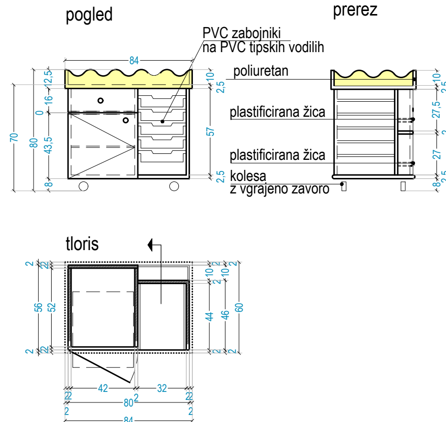
Poz. 11 SLIKARSKI VOZIČEK 84/60; H=70
