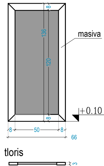
Poz. 18 OGLEDALO 50/120 pogled
