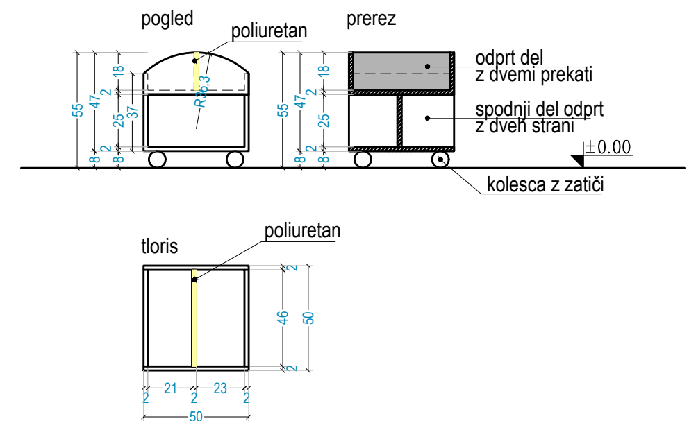
Poz. 12 VOZIČEK ZA KNJIGE 50/50, h=55
