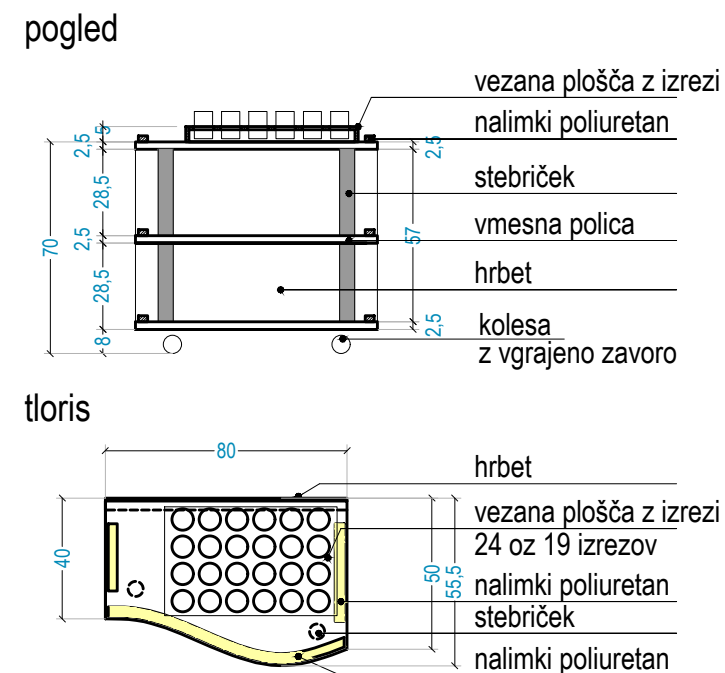
Poz. 14 SADNO ČAJNI VOZIČEK 100/50, h=70cm
