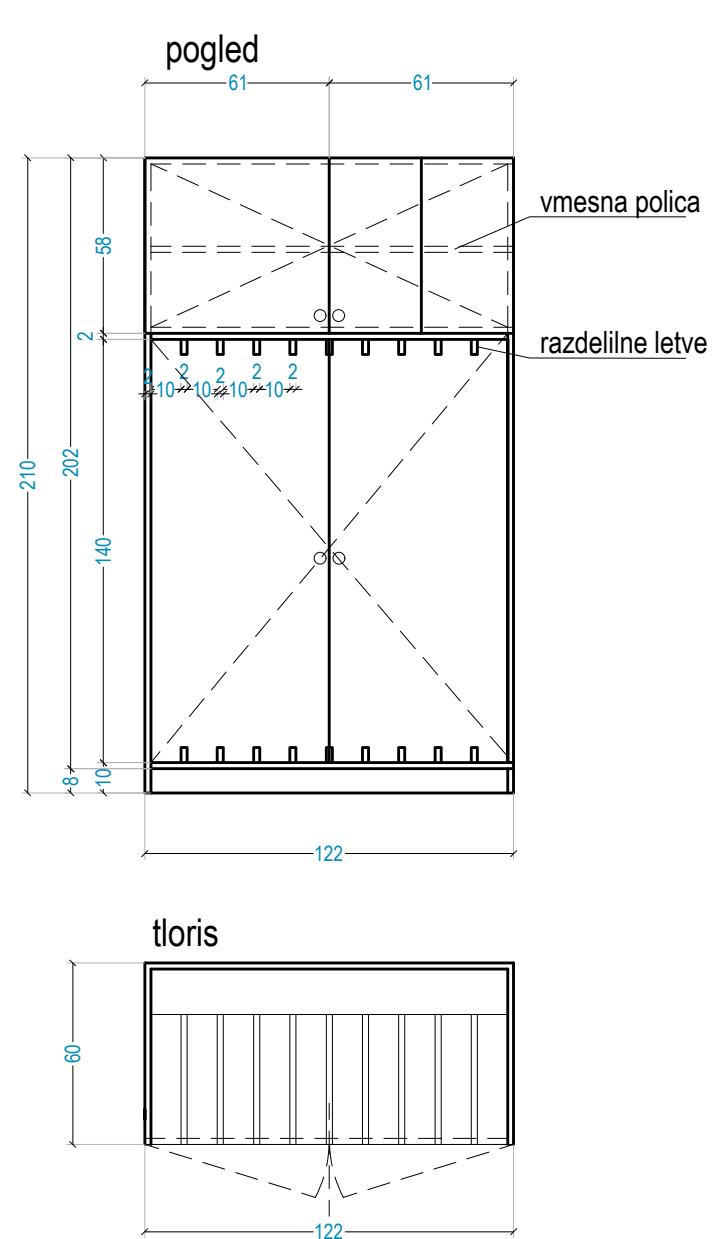
Poz.20 VISOKA OMARA ZA 10 LEŽALNIKOV 122/60, H=210cm pogled
