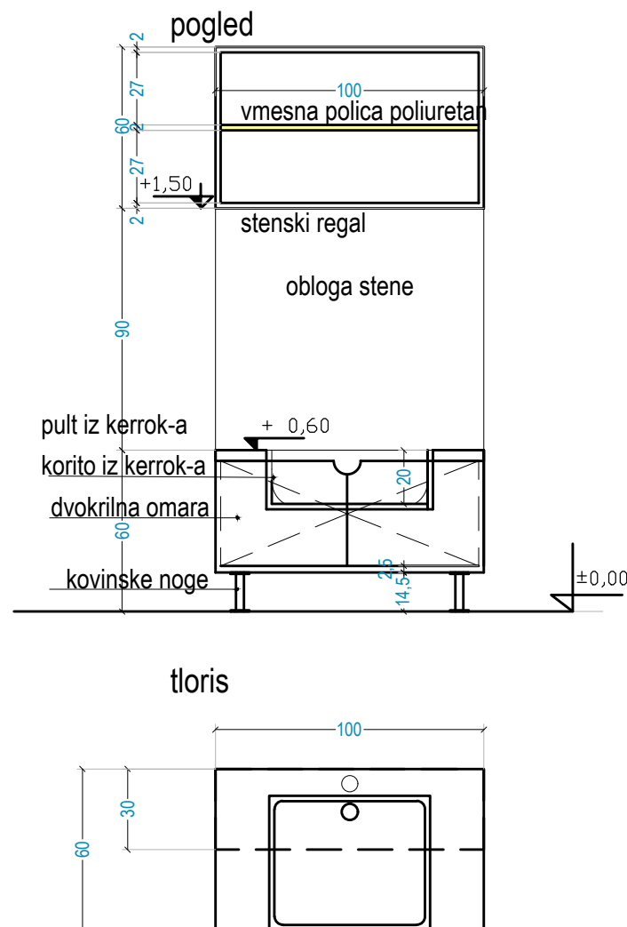
Poz. 19 KORITO V IGRALNICI 60/100cm pogled
