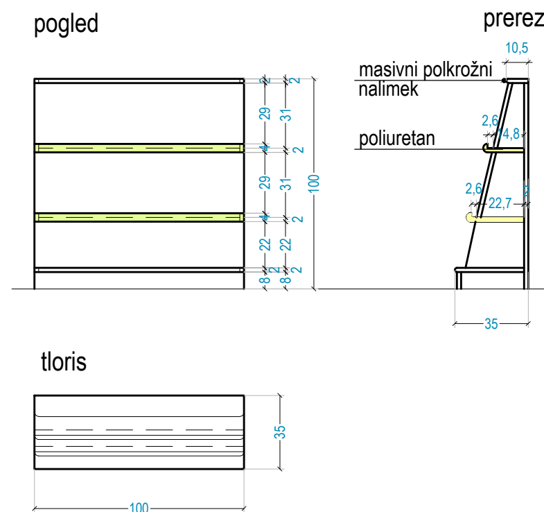
Poz. 13 KNJIŽNI REGAL 100/35; H=100
