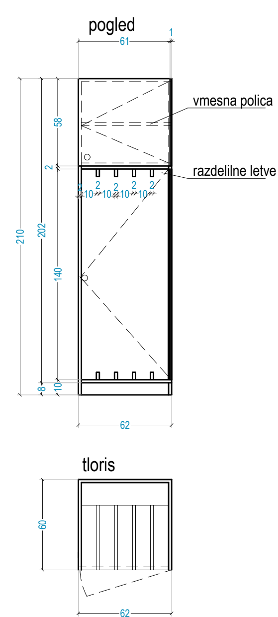
Poz.21 VISOKA OMARA ZA 5 LEŽALNIKOV 62/60, H=210cm pogled
