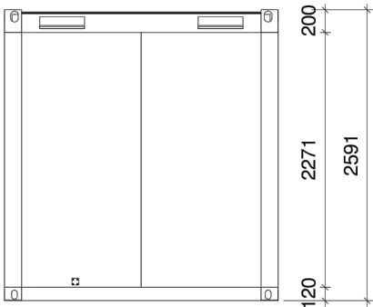
Pogled z desne 1 : 50
