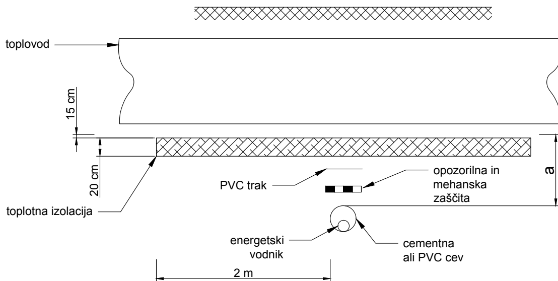
prerez A-A
