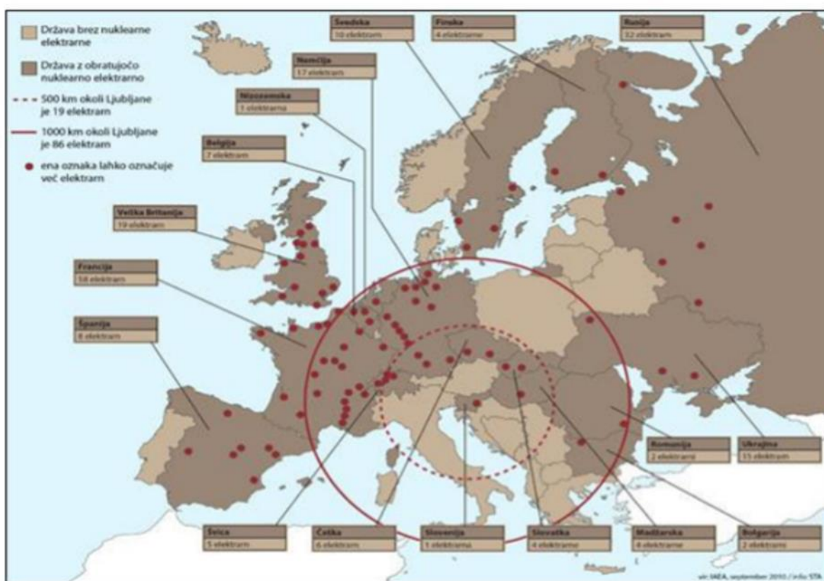
Slika 3: Jedrske elektrarne v Evropi
