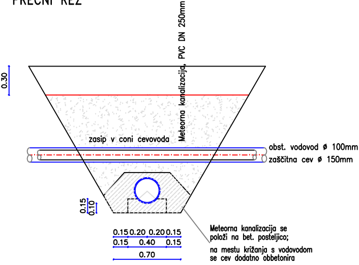
PREČNI REZ
