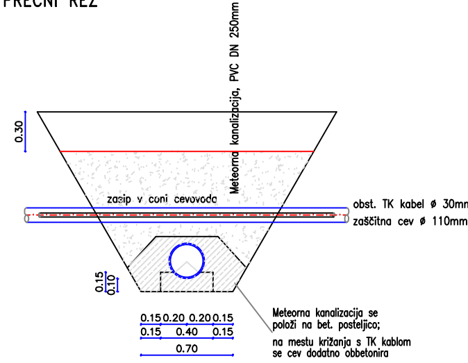
PREČNI REZ
