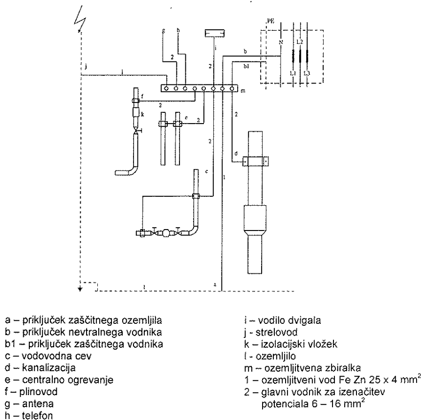
Slika 2: Izvedba glavne izenačitve potencialov za sistem TN-S
