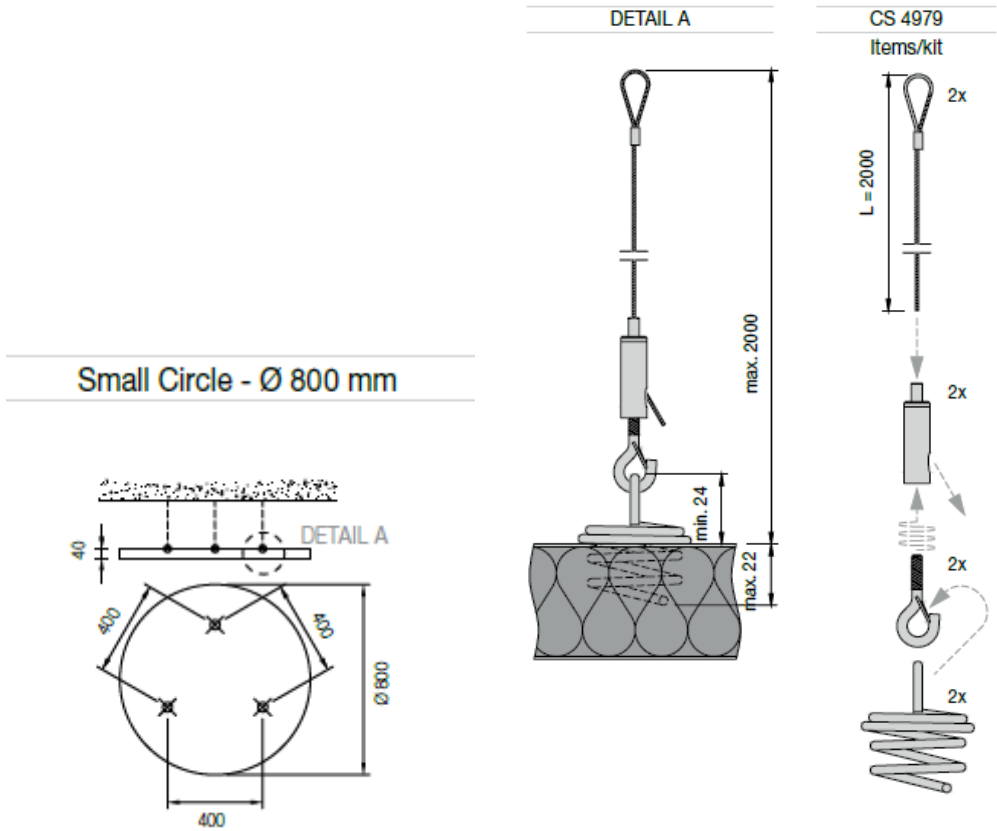
Slika 2 - sistem obešenega stropa Armstrong Optima Canopy
