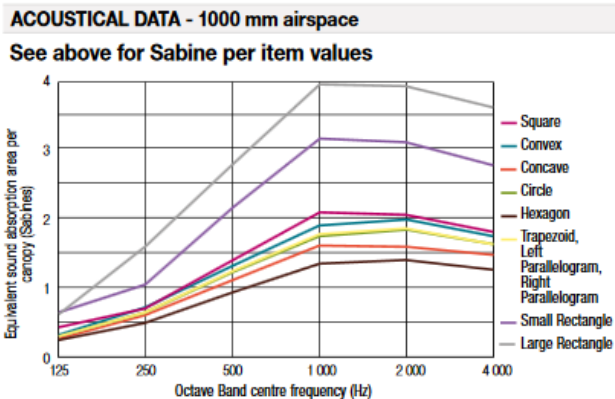
Slika 7 – akustične vrednosti sistema obešenega stropa Armstrong Optima Canopy
