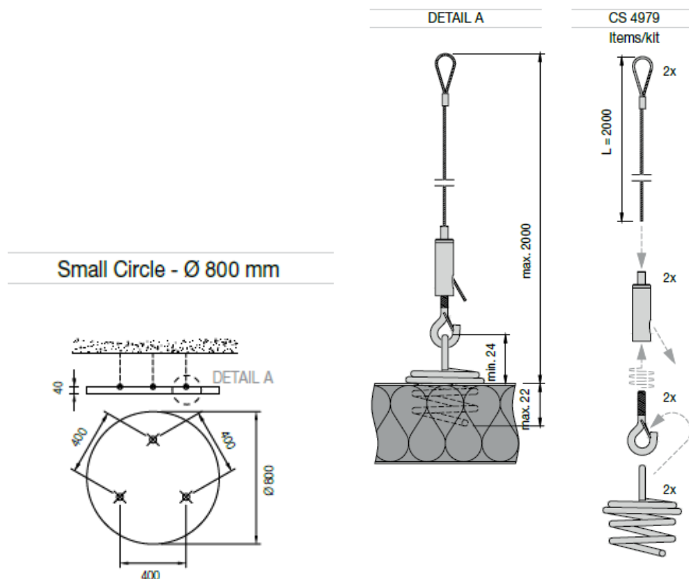
Slika 2 - sistem obešenega stropa Armstrong Optima Canopy
