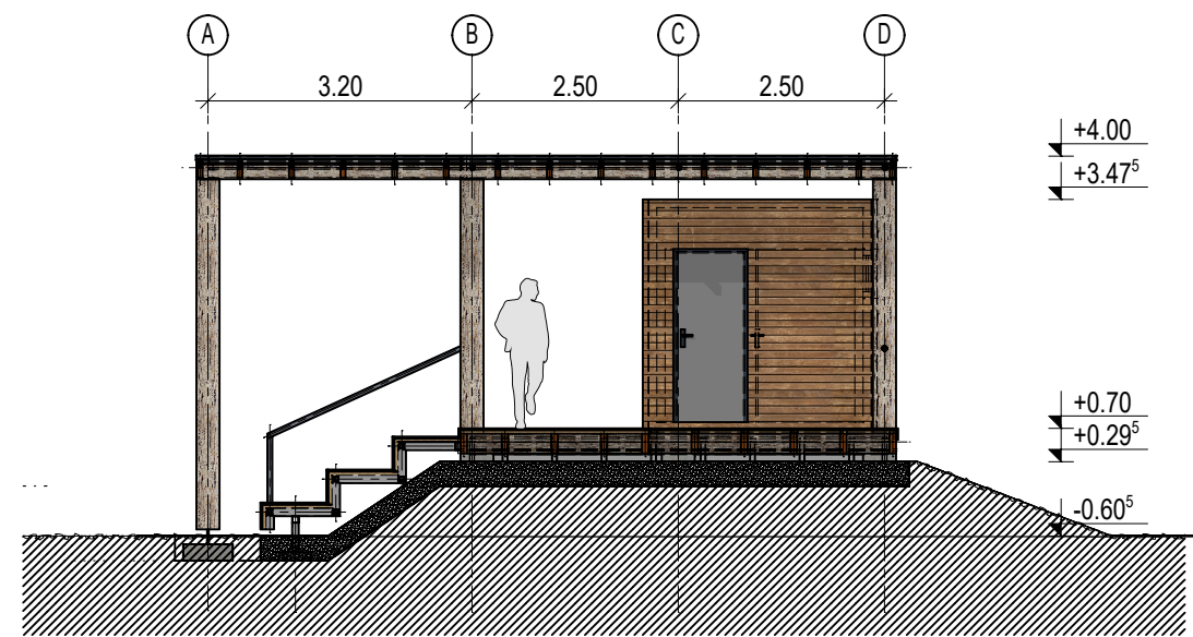
PREČNI PREREZ 4-4
