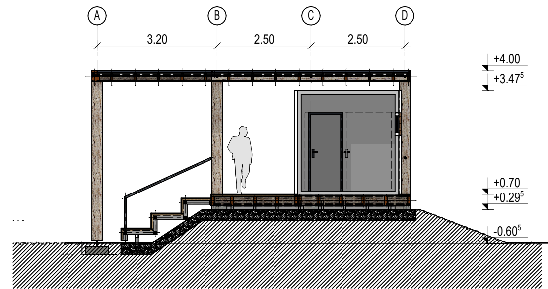
PREČNI PREREZ 3-3
