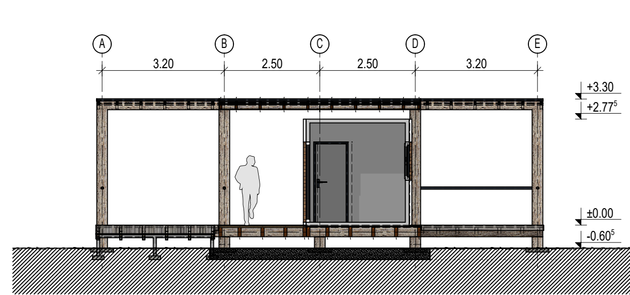
PREČNI PREREZ 2-2
