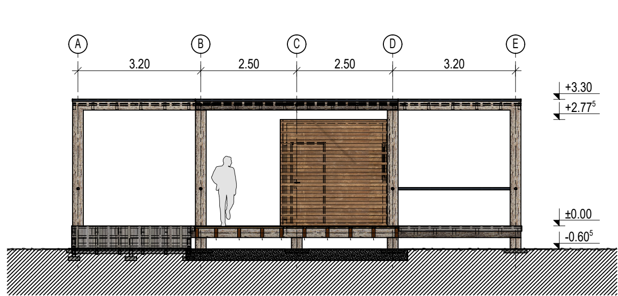
PREČNI PREREZ 1-1
