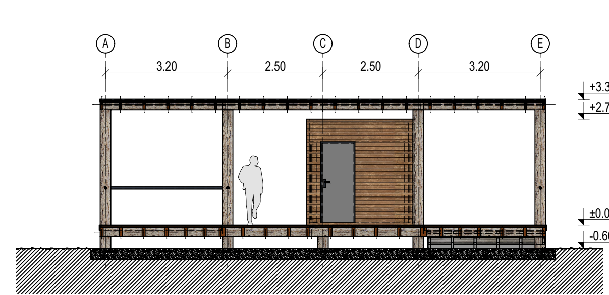
PREČNI PREREZ 8-8
