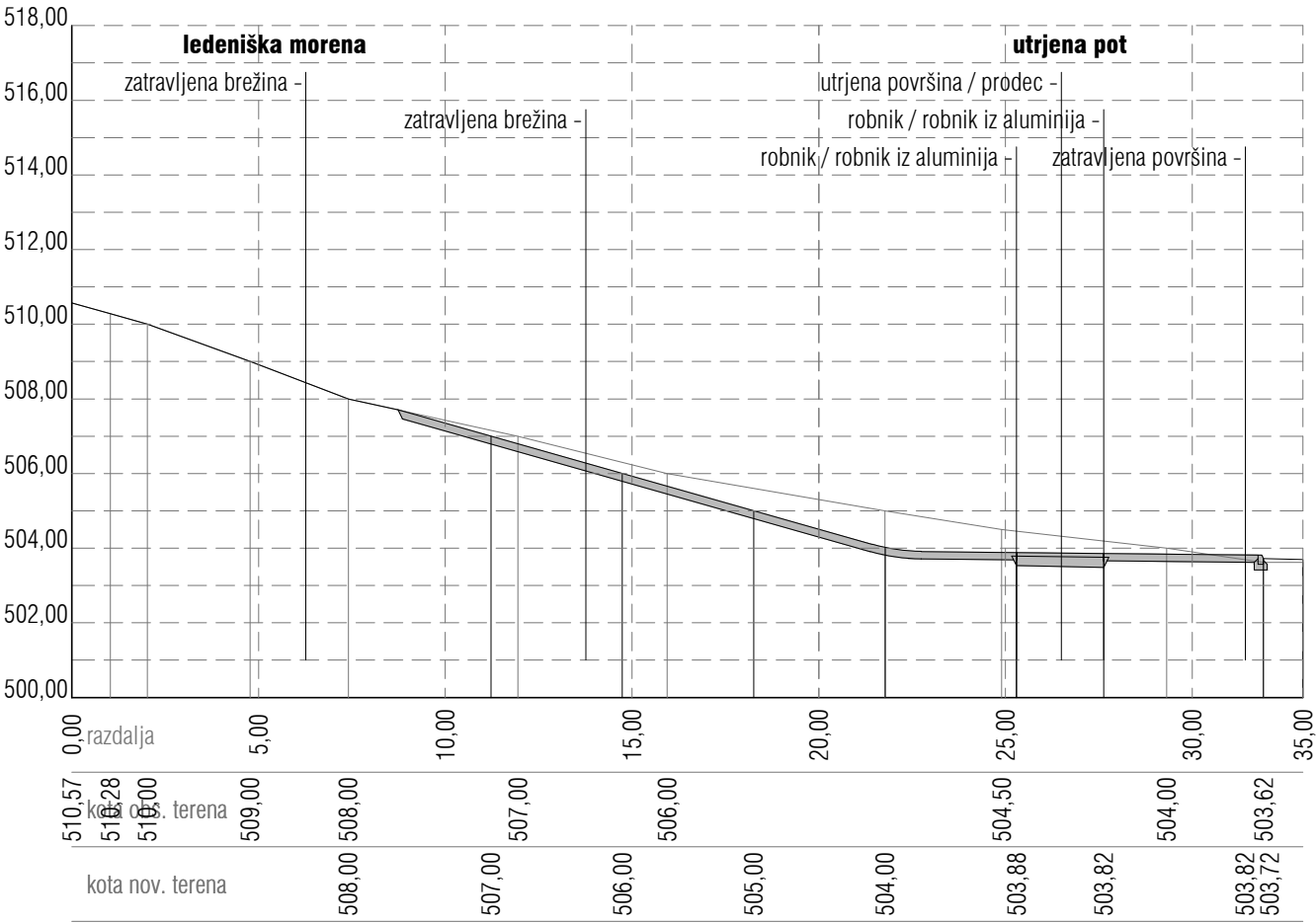
Prerez DD
