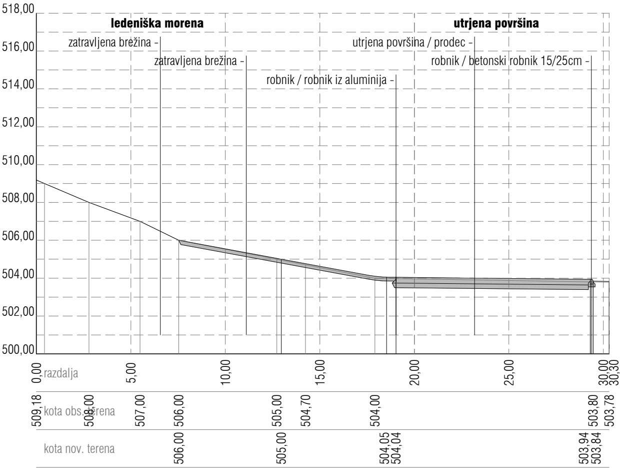
Prerez CC
