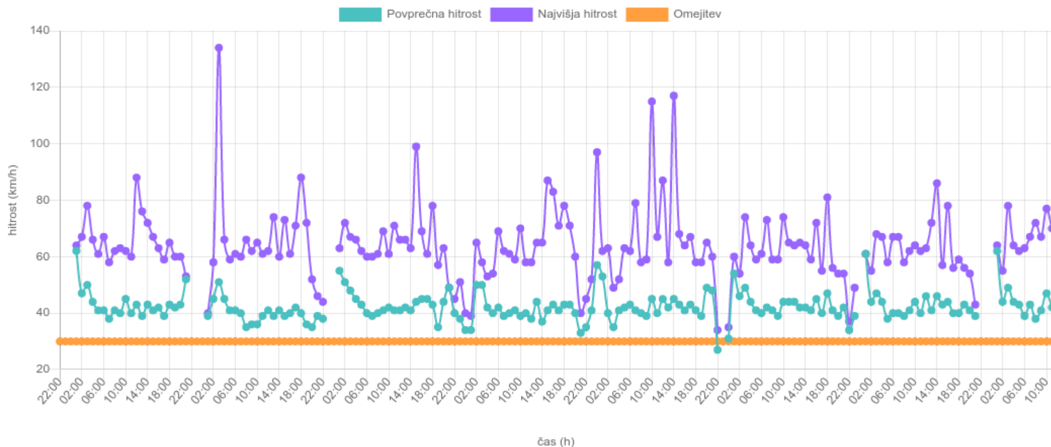
Graf 3: Povprečne in maksimalne izmerjene hitrosti v obdobju od 30.05.2023 22:00 – 07.06.2023 21:59.
