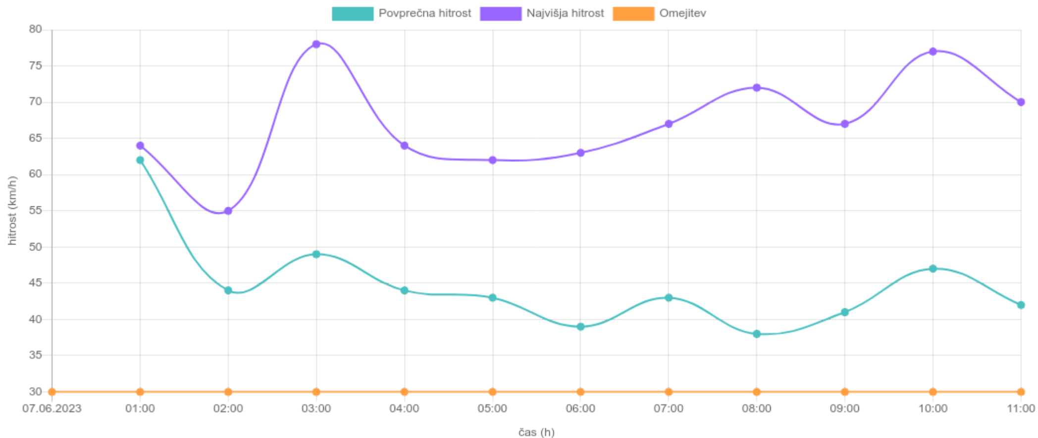
Graf 4: Povprečne in maksimalne izmerjene hitrosti na dan 07.06.2023
