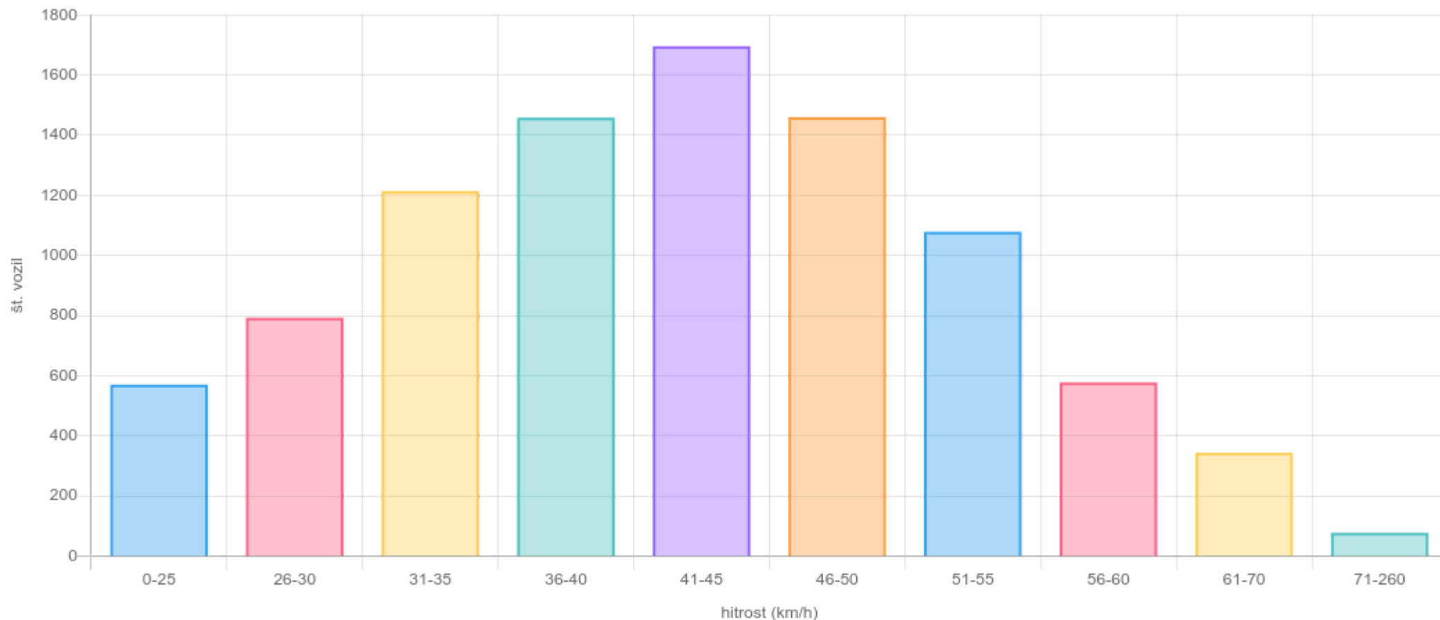
Graf 6: Porazdelitev izmerjenih hitrosti v obdobju od 30.05.2023 22:00 do 07.06.2023 21:59
