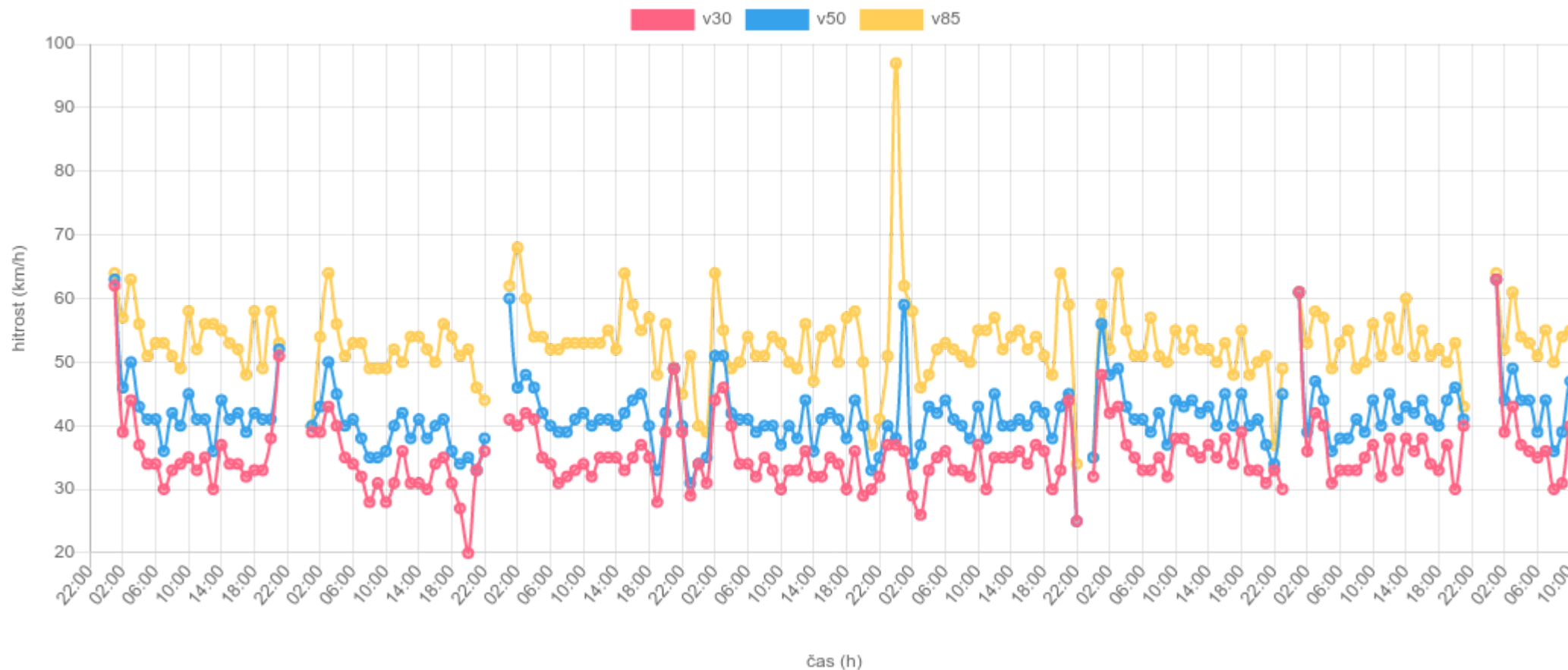
Graf 5: Percentili hitrosti (hitrost do katere je vozil določen odstotek vozil v obdobju od 30.05.2023 22:00 – 07.06.2023 21:59).
