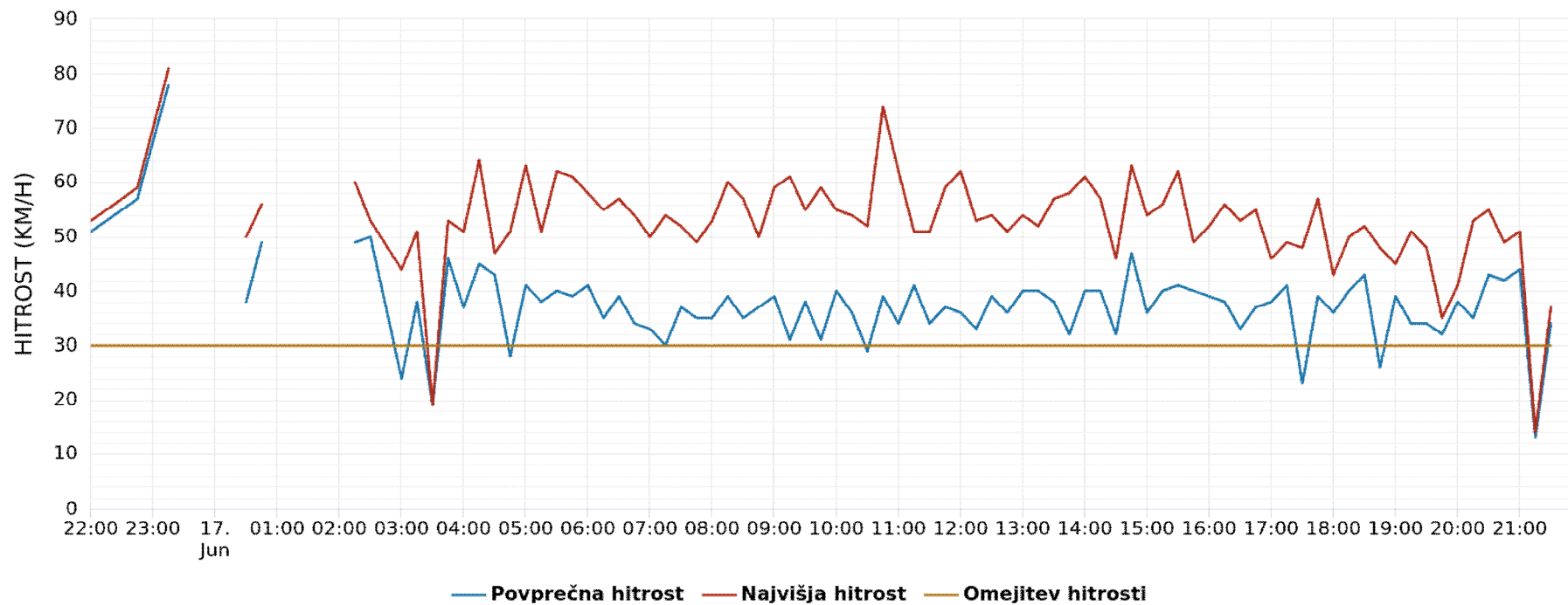
Graf 4: Povprečne in maksimalne hitrosti na dan 17.06.2019
