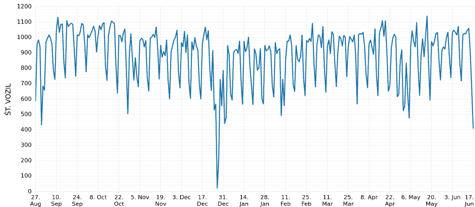
Graf 1: Št. vozil v obdobju od 27.08.2018 11:30 do 17.06.2019 11:30
