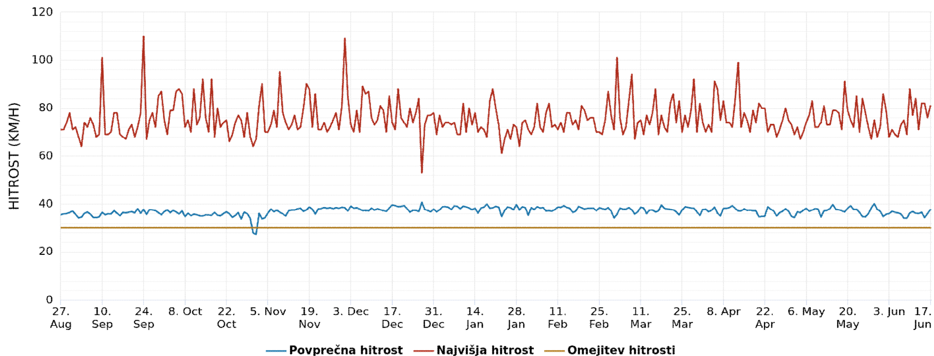
Graf 3: Zaporedje povprečnih in maksimalnih hitrosti za obdobje od 27.08.2018 11:30 do 17.06.2019 11:30
