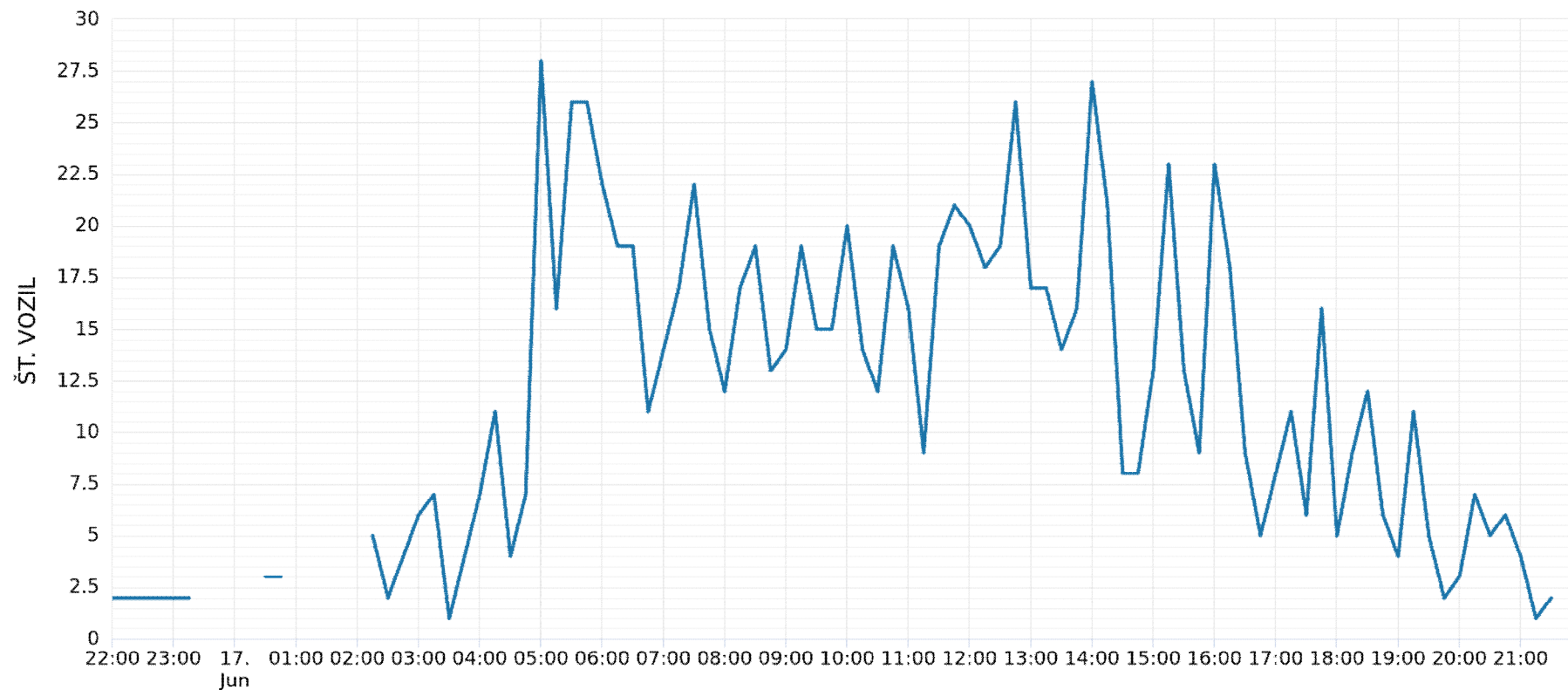
Graf 2: Podroben prikaz števila vozil v enem dnevu (17.06.2019)
