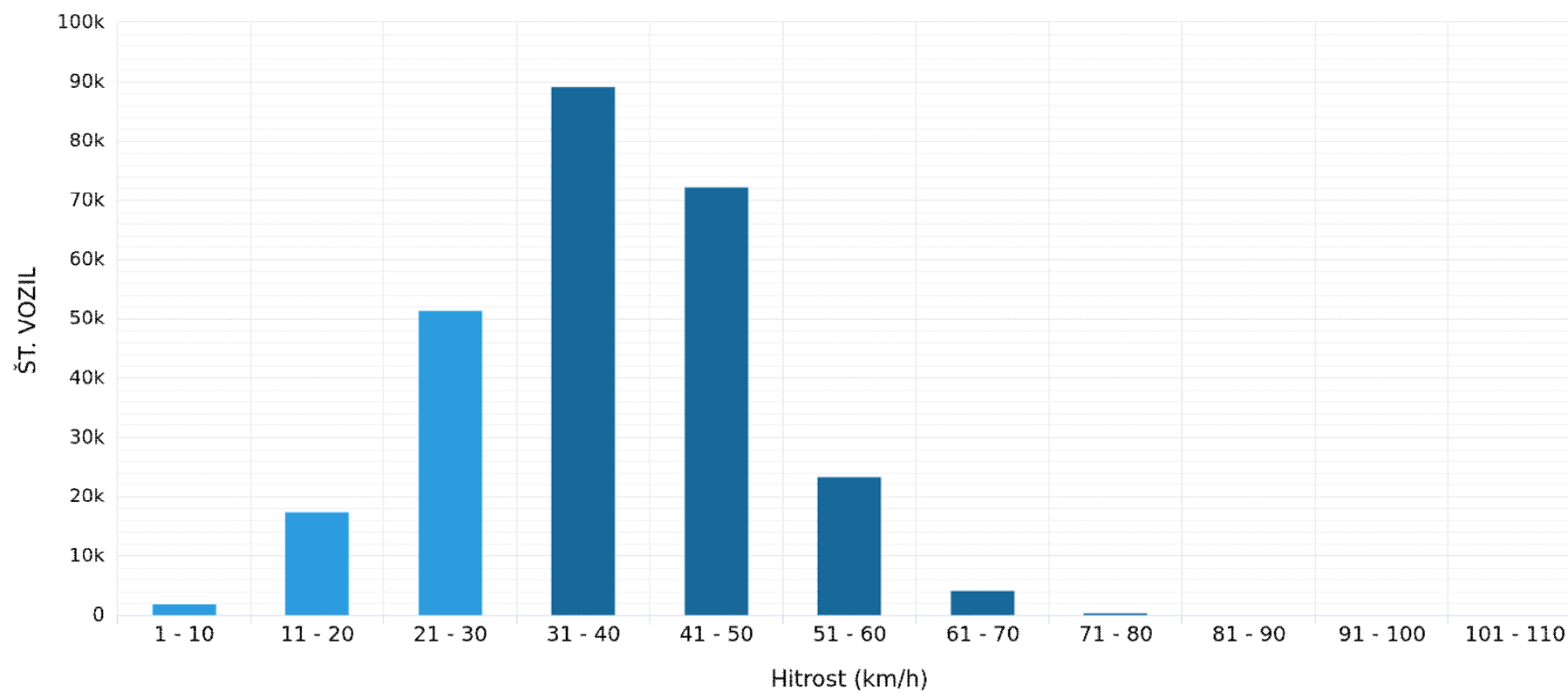
Graf 7: Porazdelitev izmerjenih hitrosti
