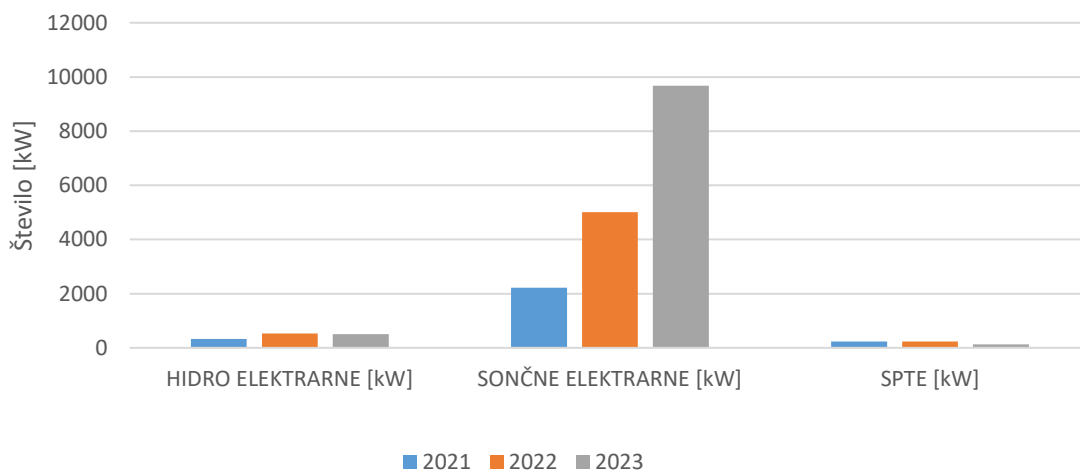
Slika 20: Priključna moč iz RV
