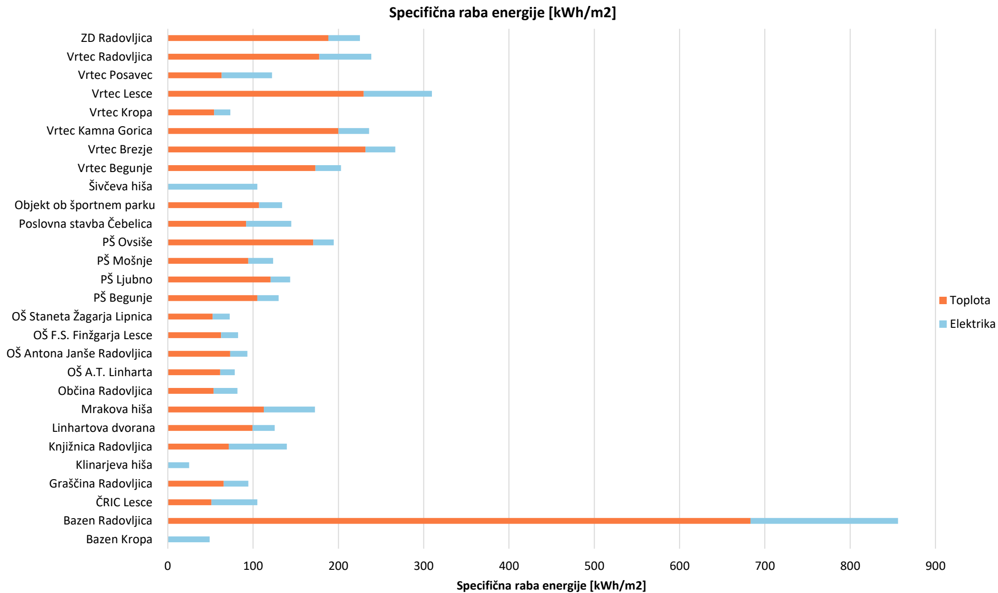
Slika 11: Specifični raba toplote in električne energije v javnih stavbah v lasti Občine Radovljica
