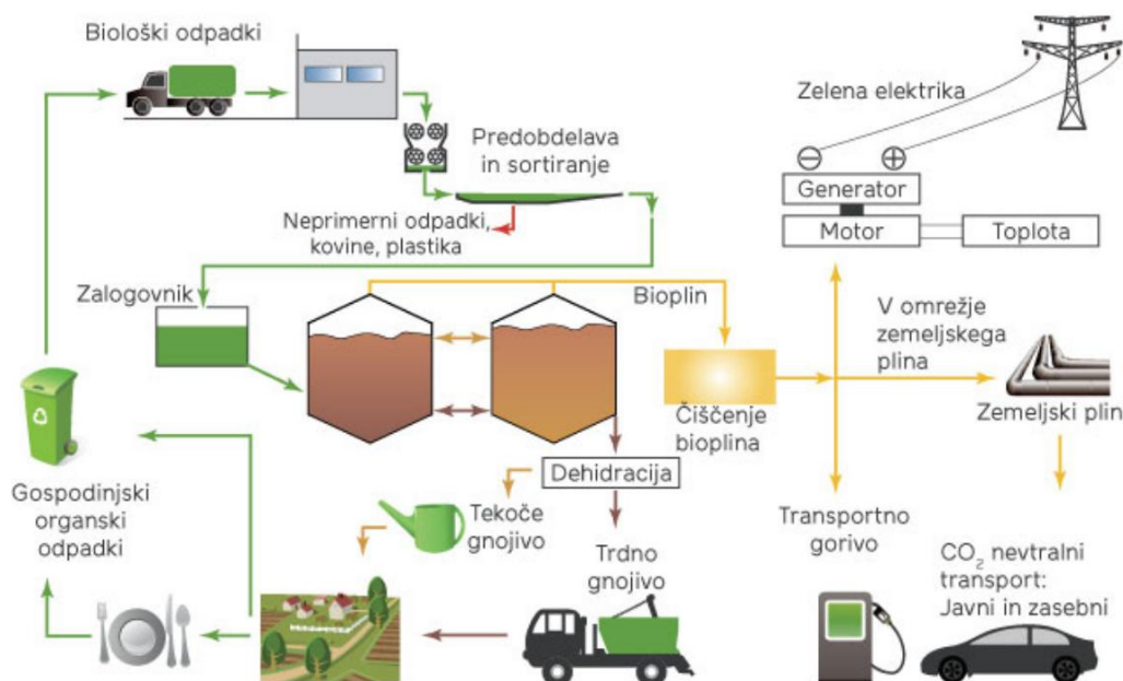
Slika 26: Proces predelave odpadkov v bioplin
