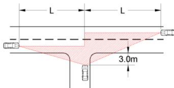
Skica 2: Primer varnostnega preglednostnega trikotnika
