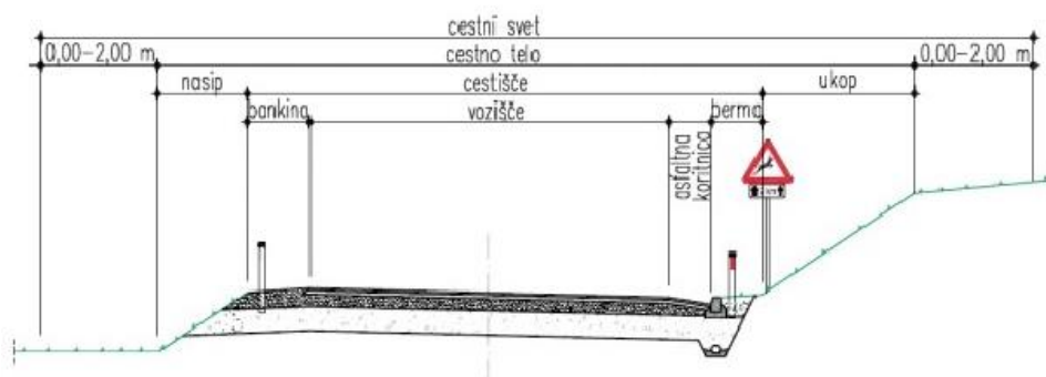
Skica 3: Sestavni deli javne ceste
