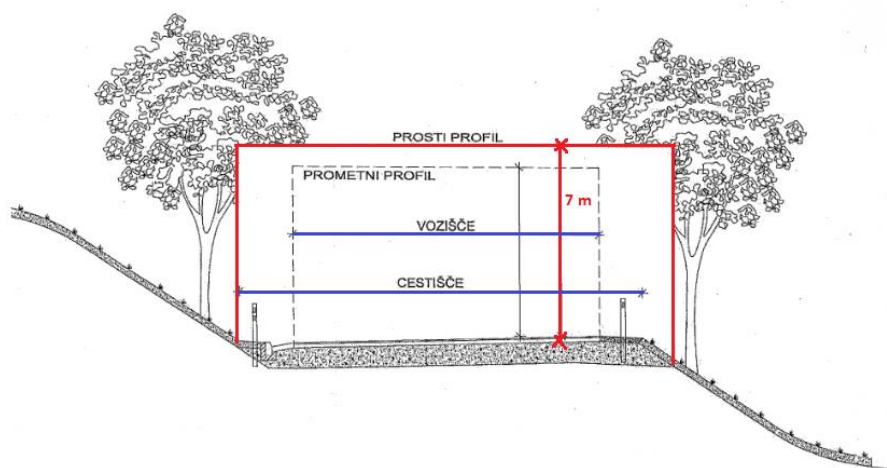
Skica 1: Zračni prostor nad cestiščem
