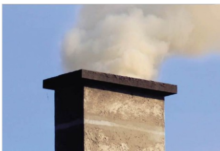
Slika 13; Temnejši ali temen gost dim na vrhu dimnika je pokazatelj zelo slabega zgorevanja (Vir: www.richtigheizen.at )
