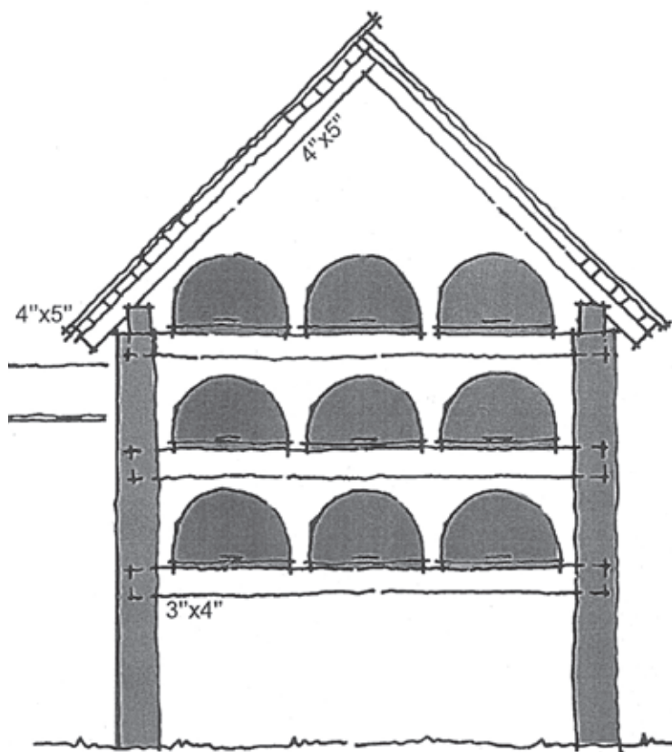
Skica čebelnjaka, avtor: Borut Juvanc
