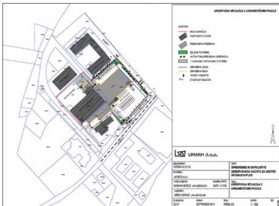
Ureditvena situacija ureditvenega načrta za širitev trgovskega centra Jager
