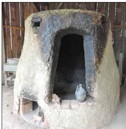
Peč za žganje keramike v Filovcih Foto: Franc Fras
