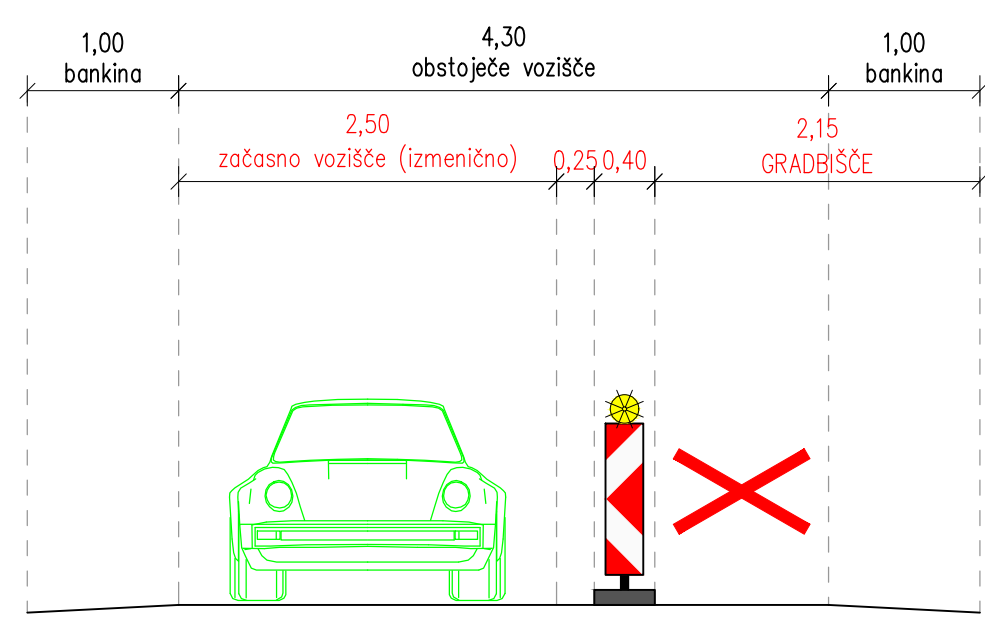
PREČNI PREREZ – FAZA 02, M 1:50 (v delovnem času in izven delovnega časa) R3-633/1098 Jereka – Jezero, v km 3,215
