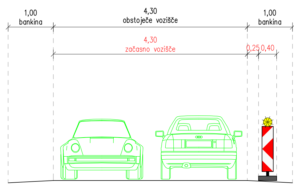
PREČNI PREREZ – FAZA 01, M 1:50 (v delovnem času in izven delovnega časa) R3-633/1098 Jereka – Jezero, v km 3,215
