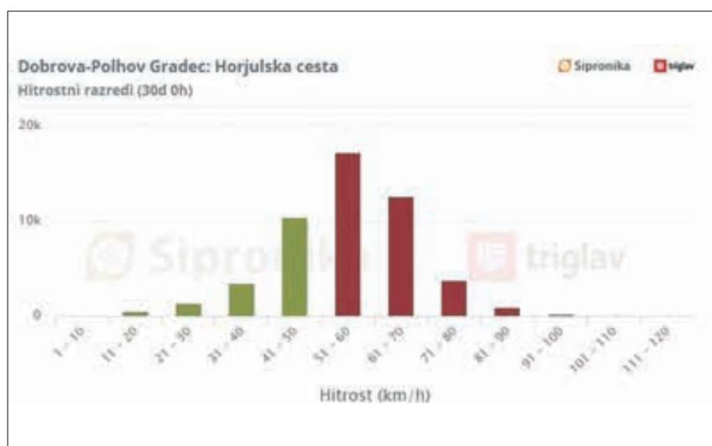
Horjulska cesta: Grafični prikaz hitrosti vožnje na dan 16. 11. 2020 za preteklih 30 dni. Rdeča barva označuje voznike, ki so prekorali omejitev hitrosti.
