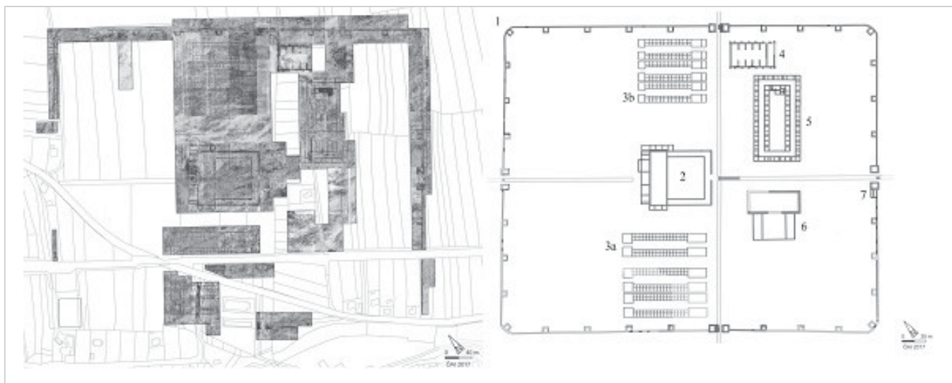
Levo rezultati geofizikalne raziskave z vidnimi arhitekturnimi ostanki (temnejše linije predstavljajo temelje zidov) ter desno načrt tabora, kot ga je interpretiral g. Groh.
