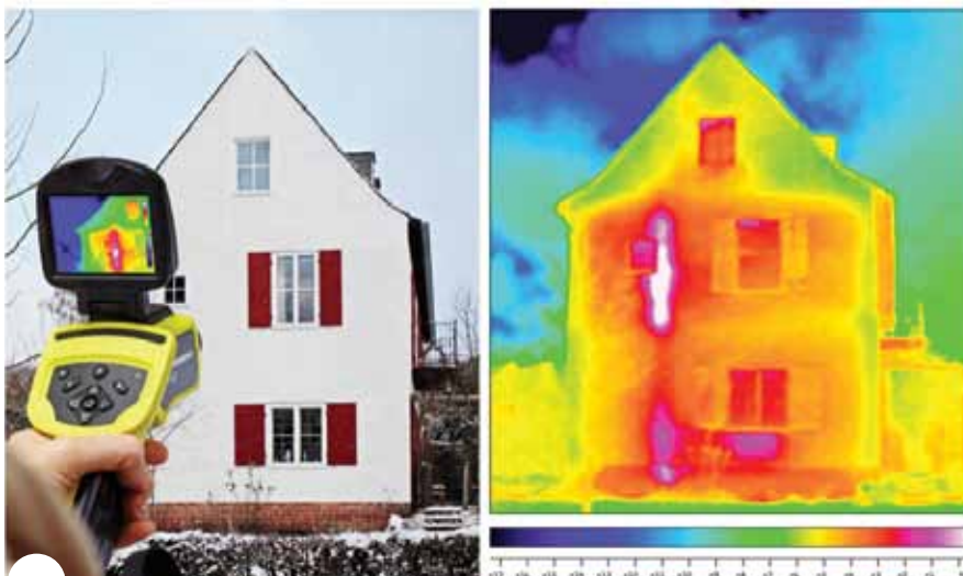
S pomočjo termografskih posnetkov se izdelava toplotna analiza stavbnega ovoja.
