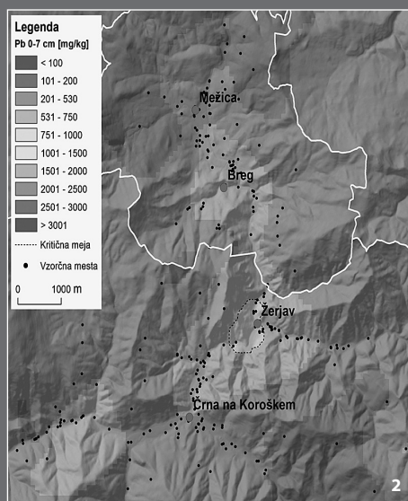
Karta onesnaženosti tal s svincem
