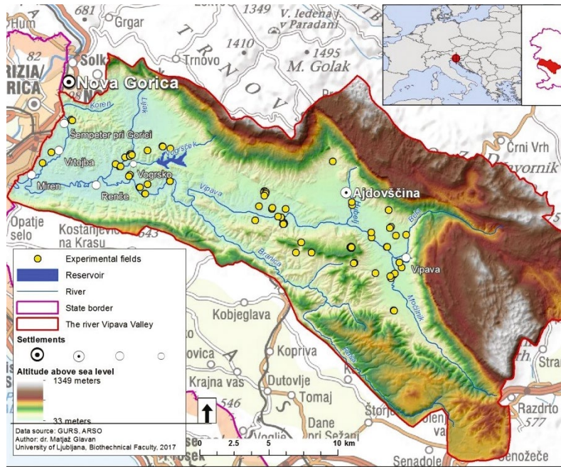
Lokacije podpisanih pogodb o sodelovanju in odvzetih vzorcih tal (Glavan M., 2016).
